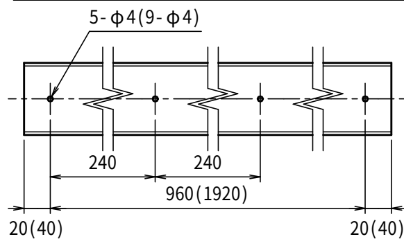
製品裏面釘穴図 ( ) は2mの意。
